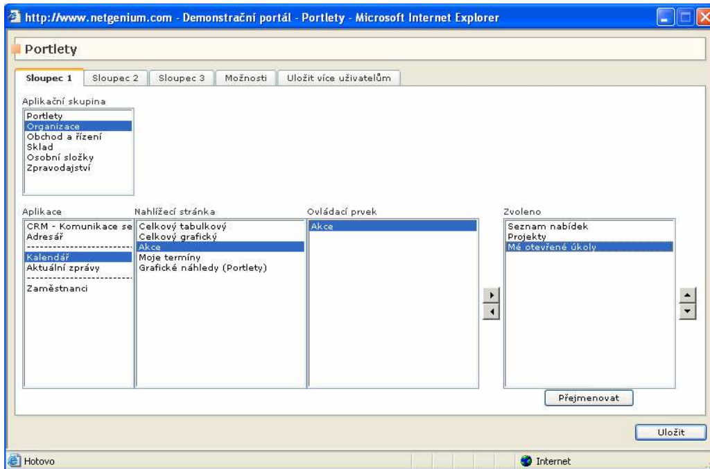
Obrázek 2.5: Nastavení portletů
